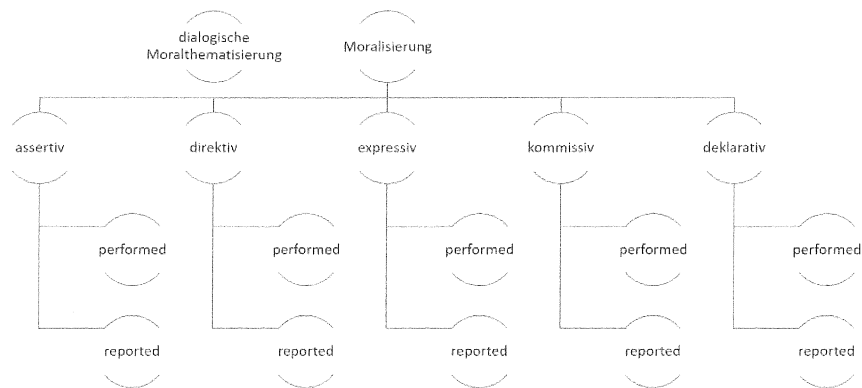
Abb. 2: Annotationsschema
